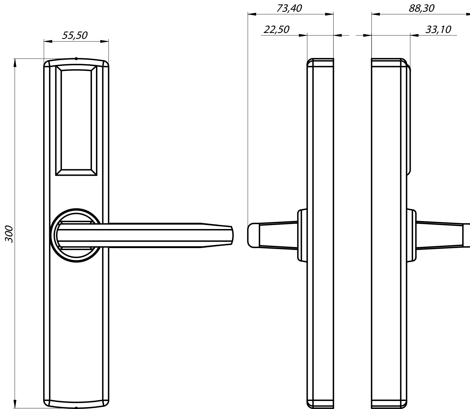
Rysunek złożeniowy szyldu elektronicznego LOB 5500 Adel
